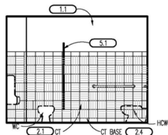
03 MENS SCALE: 1/4"=1'-0"
