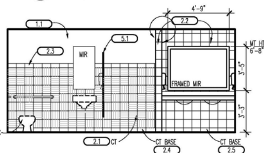
04 MENS SCALE: 1/4"=1'-0"
