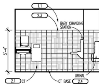
01 MENS SCALE: 1/4"=1'-0"
